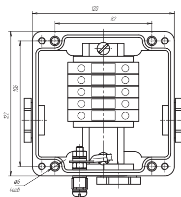
Коробка с винтовым клеммным блоком
