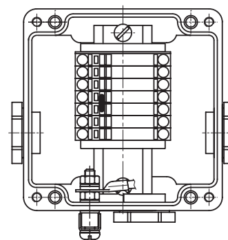
Коробка с пружинным клеммным блоком
